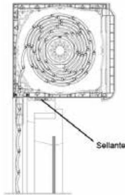
Figura 56. Detalle de unión de carpintería a cajón de persiana indicando posición del sellante
