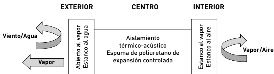
Figura 21. Esquema de aislamiento de la junta
