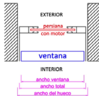
Figura 50. Esquema sección horizontal de ventana con persiana con motor con solución simétrica y muro de cerramiento de gran espesor
