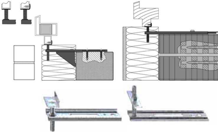
Figura 20. Consolas
