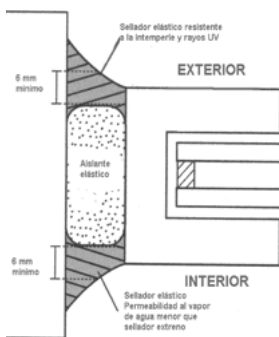
Figura 22. Sellado a testa
