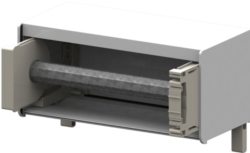
Figura 43. Sistema de testereros que posibilitan extracción del eje
