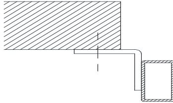
Figura 11. Anclaje sobrepuesto
