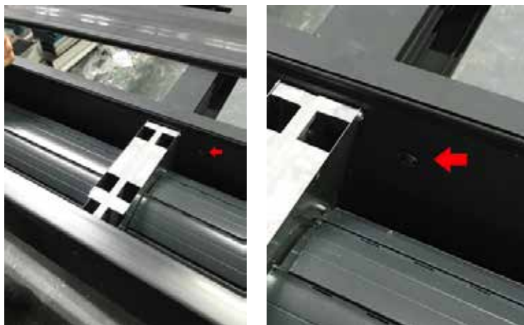
Figura 62. Detalle atornillado visto interiormente. Cuidado que la cabeza del tornillo no perforo el cajón.
