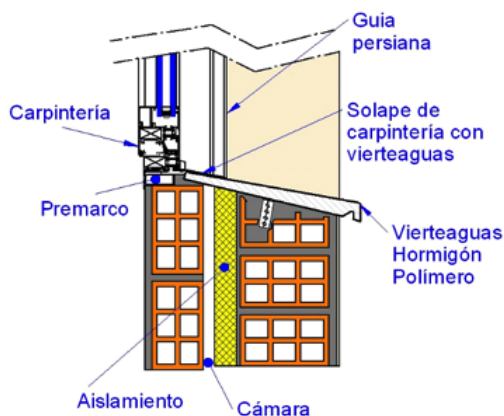
Figura 85. Esquema vierteaguas
