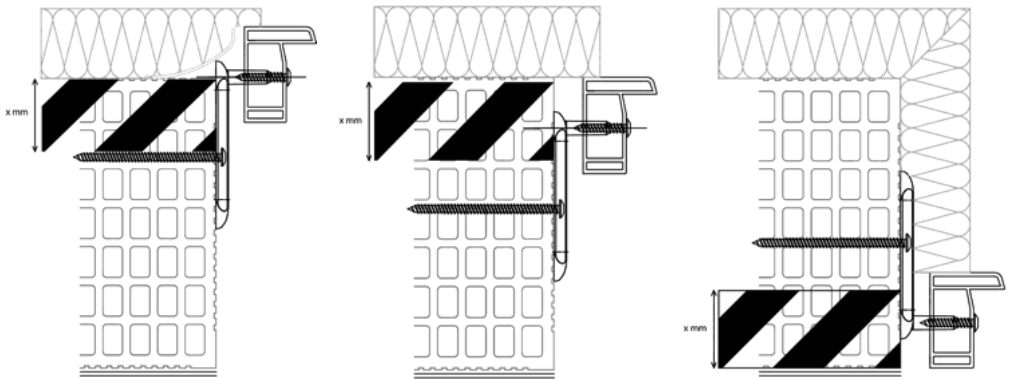
Figura 19. Fijación desplazada
