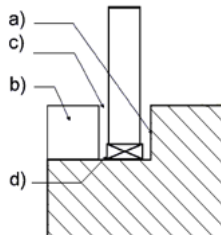
Figura 25. Definición de un galce de acristalamiento
